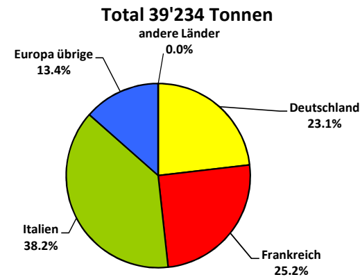
Käseimporte nach Ländern, Januar bis September 2013
